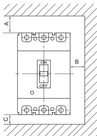
断路器在金属柜体间的绝缘距离
