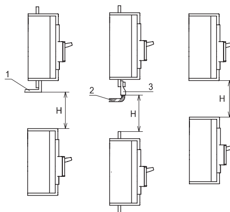
1. 连接 - 无绝缘 2. 绝缘电缆 3. 电缆端子
